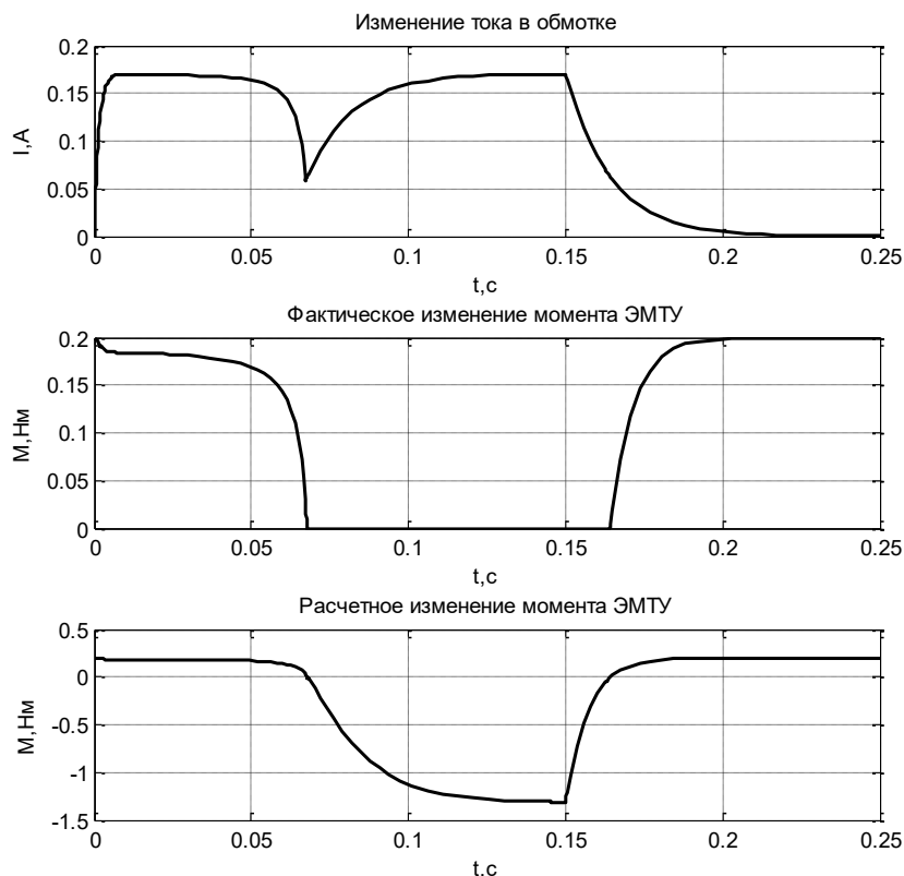
Рисунок 6 – Переходные процессы при включении и последующем отключении питания обмотки ЭМТУ
